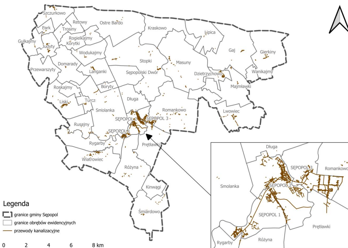
Ryc. 23. Sieć kanalizacji sanitarnej na terenie gminy Sępól
