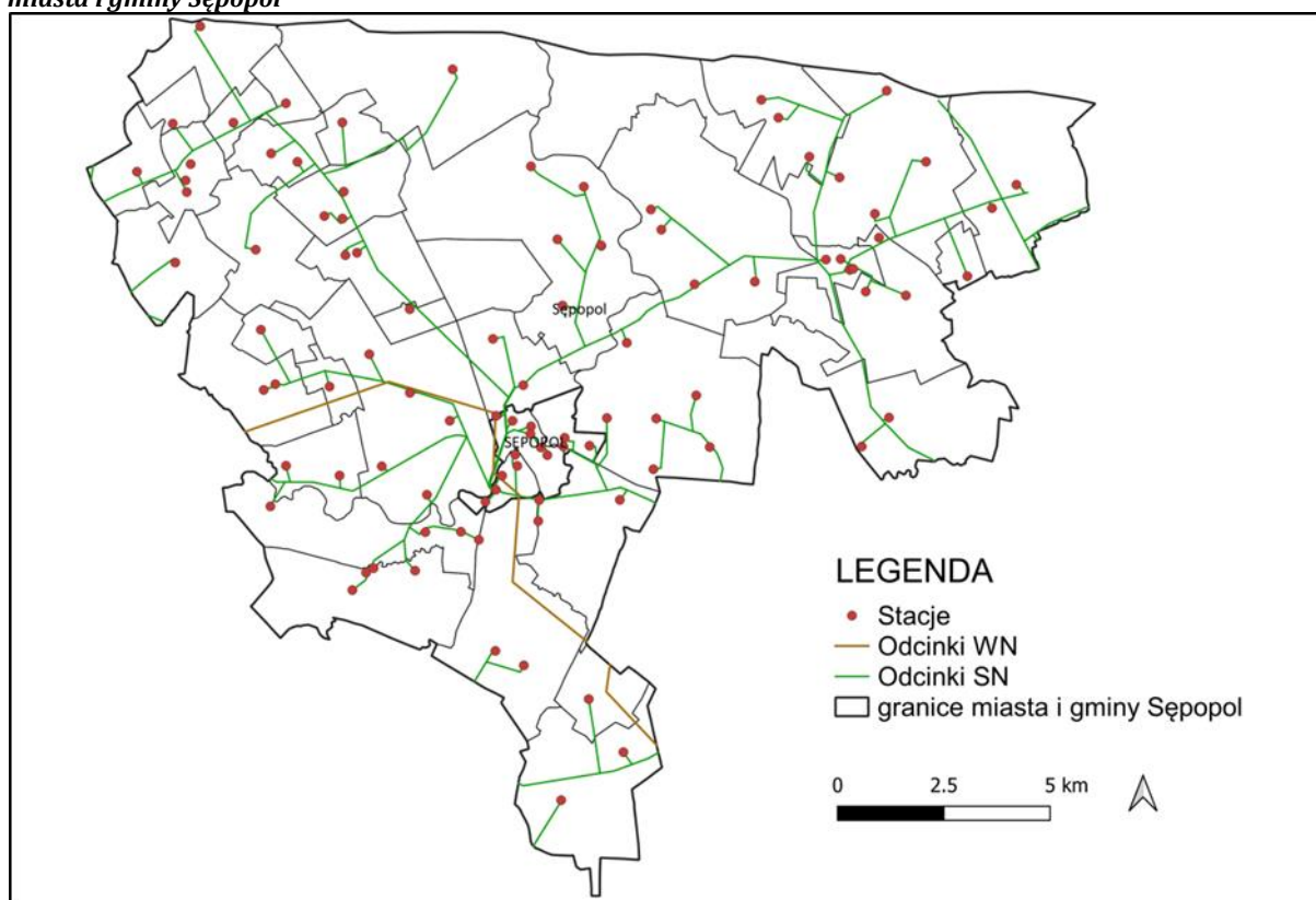
Ryc. 23. Przebieg linii wysokiego i średniego napięcia oraz lokalizacja stacji transformatorowych na terenie miasta i gminy Sępól
