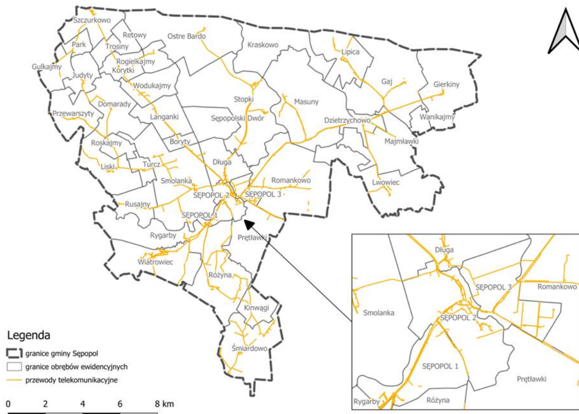
Ryc. 25. Sieć telekomunikacyjna na terenie gminy Sępól
