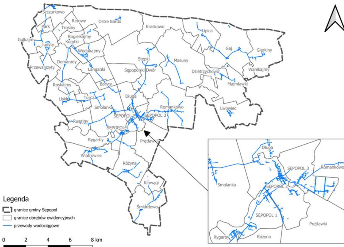
Ryc. 21. Sieć wodociągowa na terenie gminy Sępól
