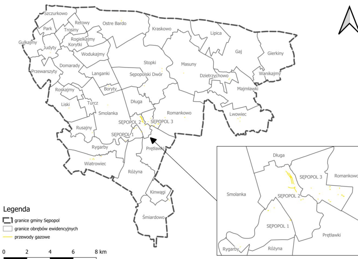
Ryc. 25. Sieć gazowa na terenie gminy Sępapol
