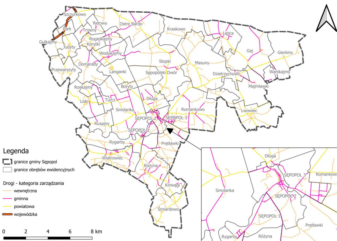
Ryc.25.Schemat sieci drogowej na terenie gminy Sępól
