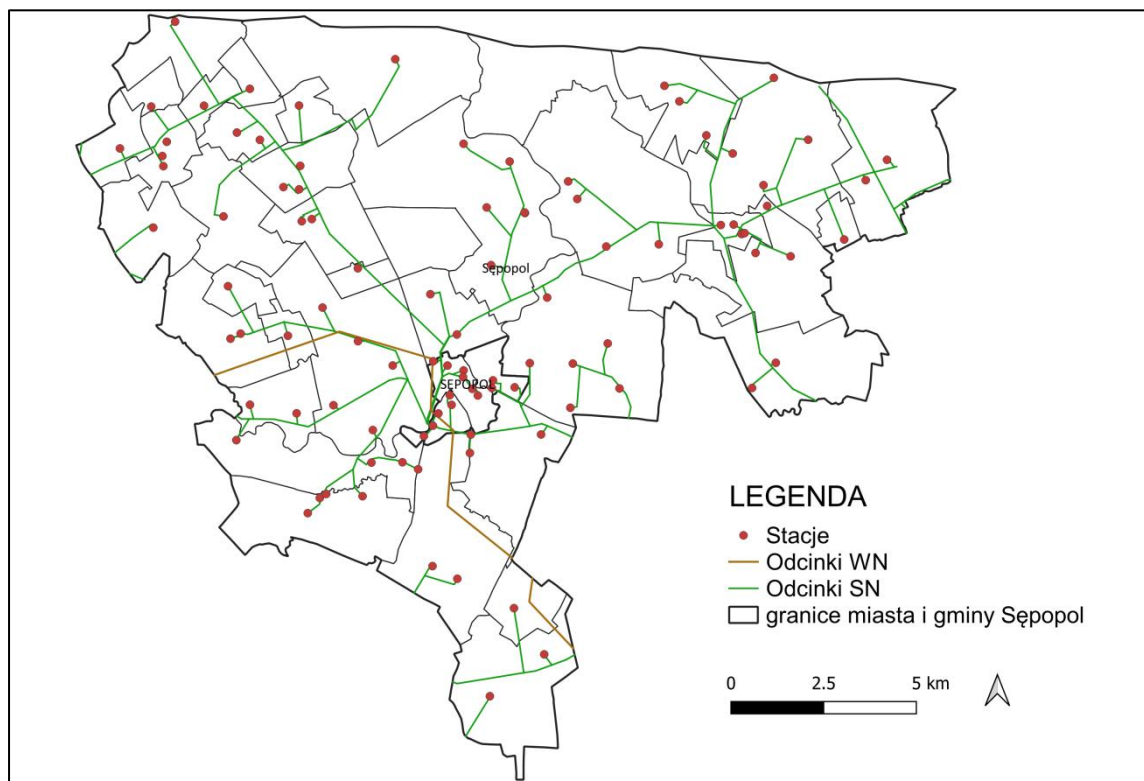
Ryc. 26. Przebieg linii wysokiego i średniego napięcia oraz lokalizacja stacji transformatorowych na terenie miasta i gminy Sępólno.
