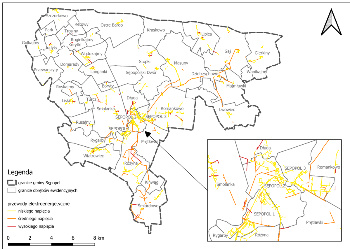
Ryc. 27. Sieć elektroenergetyczna na terenie gminy Sępól
