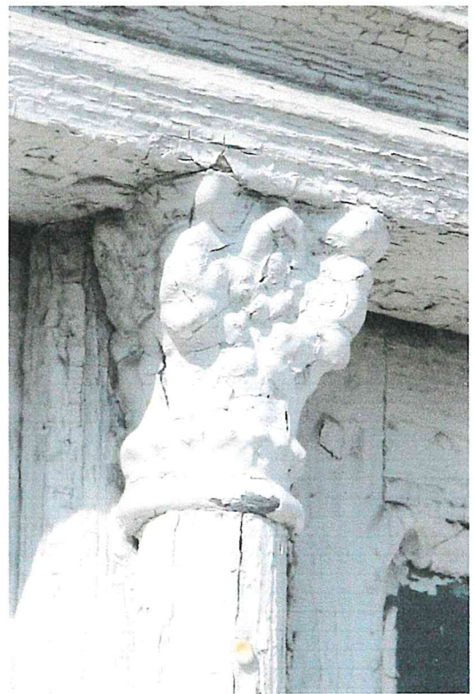
Oryginalne okno wyposażone jest w półwałki na listwach przymykowych, cynowe kapitele i profilowane ślemię.
